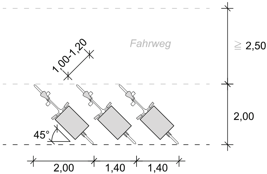
Schrägaufstellung 45^\circ
