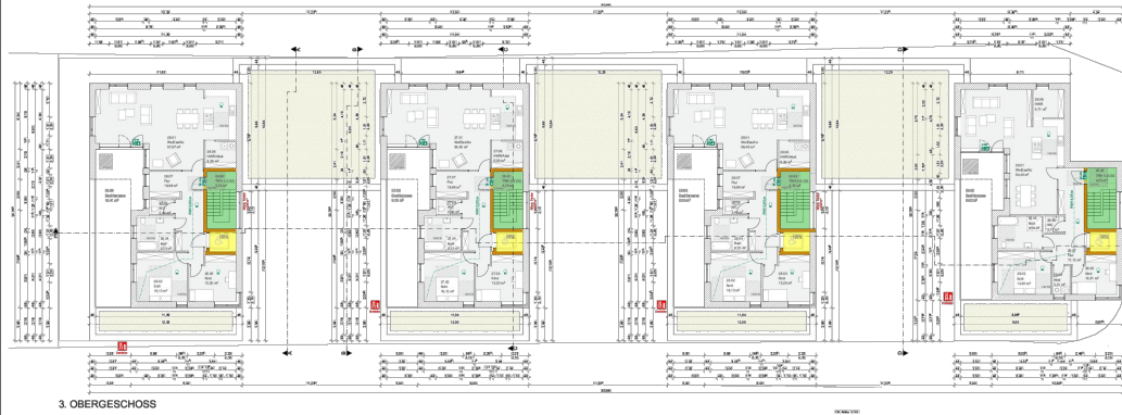
3. OBERGESCHOSS
