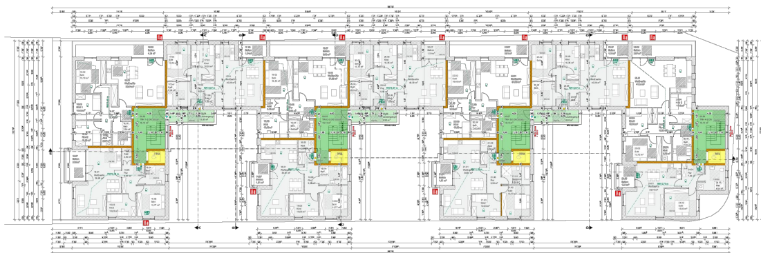
2. OBERGESCHOSS
